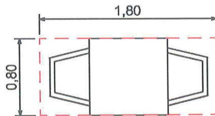
MÓDULO 3. 2 SILLAS - 1 MESA S = 1,44 m 2
